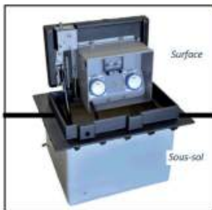
Borne électrique (1)
